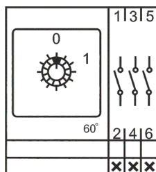
FUNKCJA 0-1, 3P
